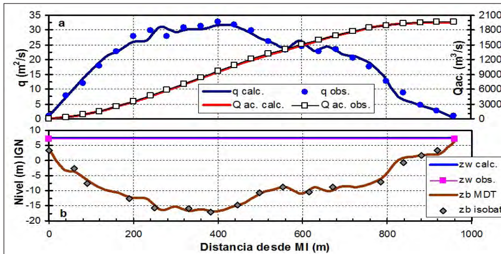
Figura 5.- Simulación S4-C1R5, Q=19570 m³/s. Sección transversal km 429. a) Comparación de la distribución de caudales específicos q calculados y observados y correspondiente curva de caudales acumulados Qac. b) Nivel hidrométrico calculado y observado; nivel del lecho del MDT y nivel del lecho observado a partir de relevamiento batimétrico.
